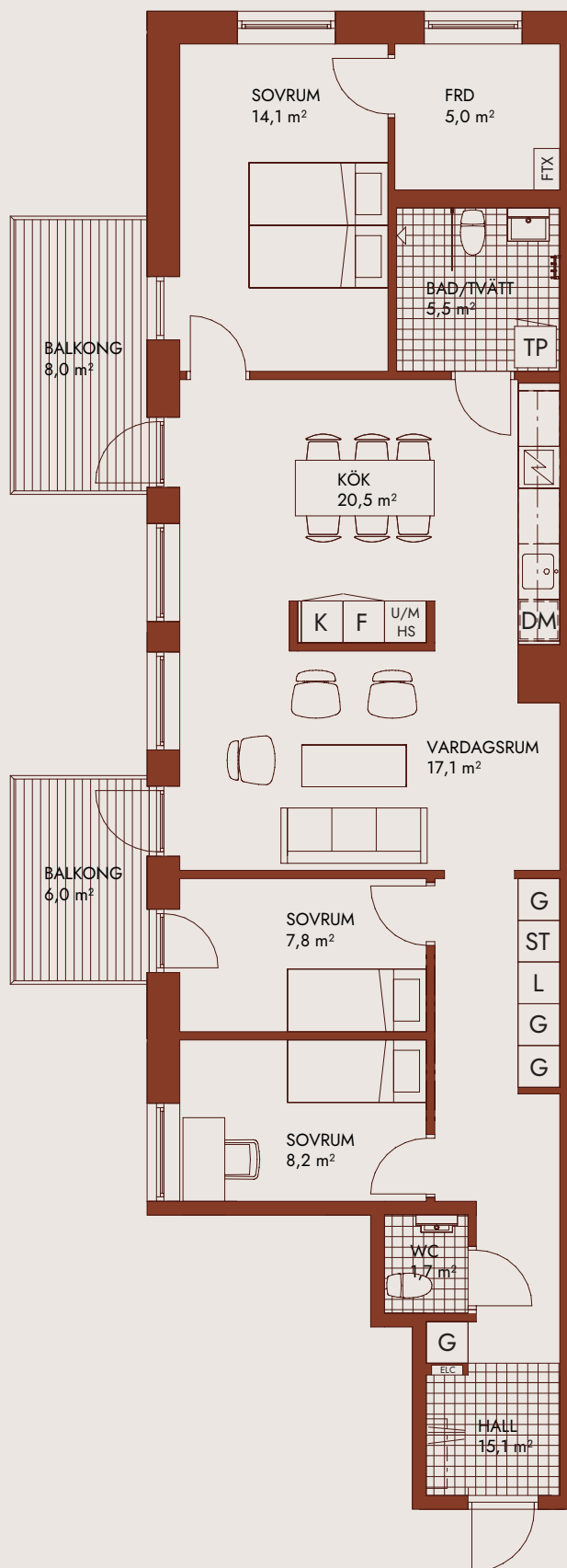
VÅNINGSPÄN
