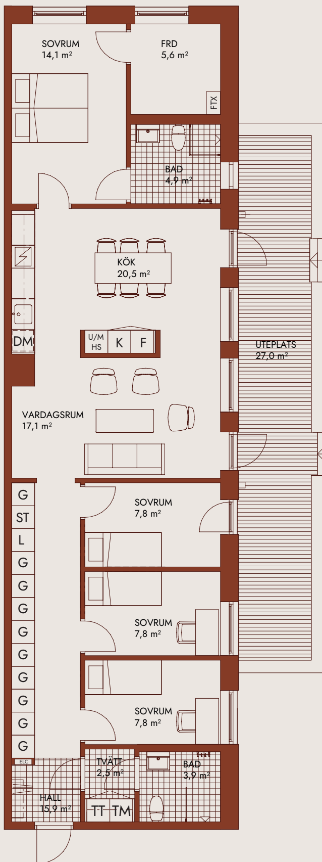
VÅNINGSPLAN
